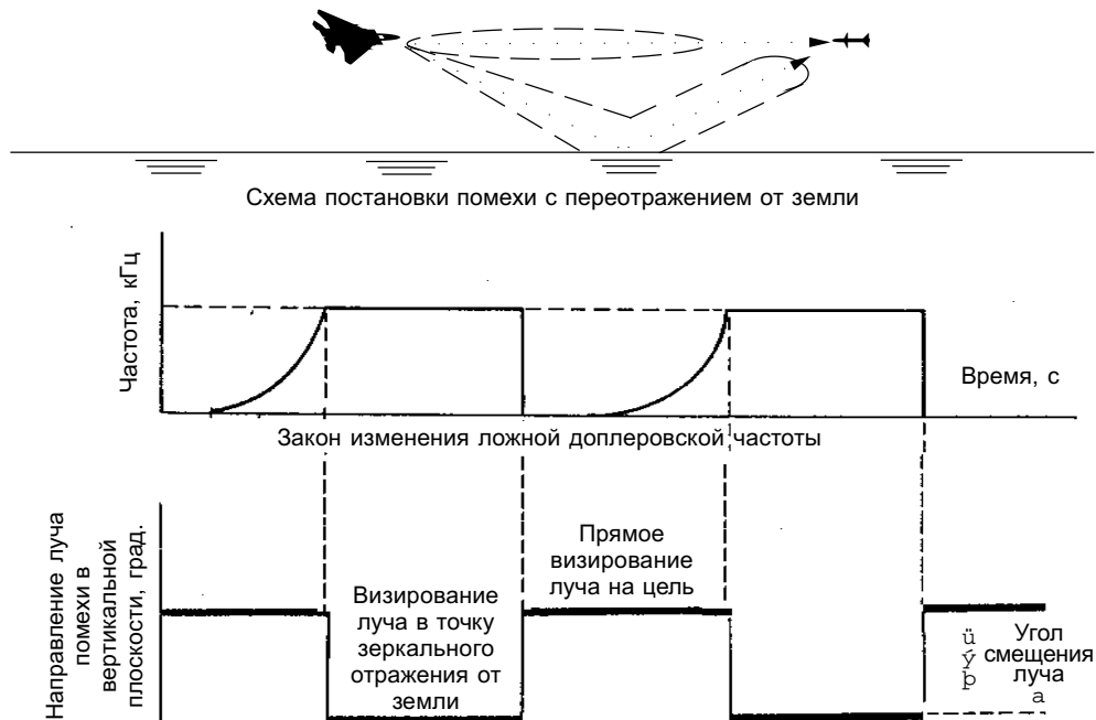
Рис. 5. Процесс постановки увода строба скорости доплеровской радиолокационной ГСН при использовании коммутации прямого и отраженного от земной поверхности лучей помехового сигнала
