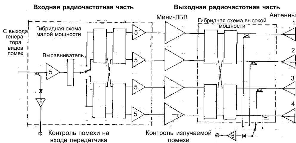
Рис. 7. Усилительная часть передатчика помех диапазона 6,5 – 18 ГГц на четырех двухрежимных мини-ЛБВ с гибридной схемой коммутации четырех антенн на борту ЛА: 1, 2, 3, 4 – номера антенн; 5 – твердотельный усилитель мощности; 6 – видеусилитель схемы контроля излучения помехи
