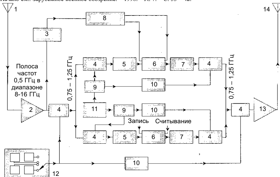
Рис. 1. Структурная схема DRFM диапазона 8 – 16 ГГц: 1 – приемная антенна; 2 – предварительный усилитель приемника; 3 – детектор; 4 – смеситель; 5 – преобразователь «аналог-цифра»; 6 – быстродействующее магнитное ЗУ с произвольным доступом; 7 – преобразователь «цифра-аналог»; 8 – программирующее устройство; 9 – разветвитель; 10 – схема развязки; 11 – опорный генератор 1 ГГц; 12 – блок опорных генераторов первого гетеродина; 13 – усилитель мощности; 14 – передающая антенна
