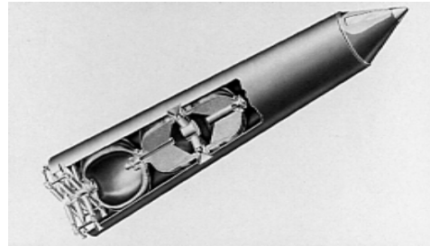
Рис. 2. Общий вид ступеней перехвата – с железобразной (слева) и с твердотопливными двигательными установками маневрирования и пространственной ориентации
