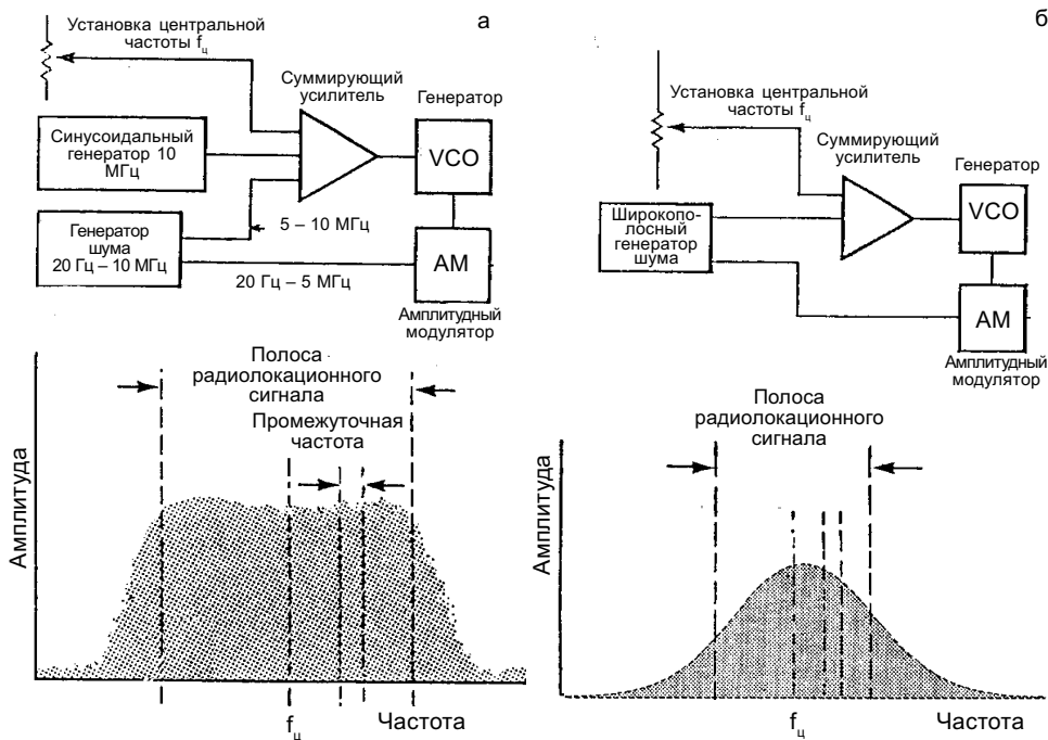
Рис. 4. Структурные схемы и спектры источников шумового помехового сигнала: а – усовершенствованной конструкции (высокочастотный источник); б – обычной
